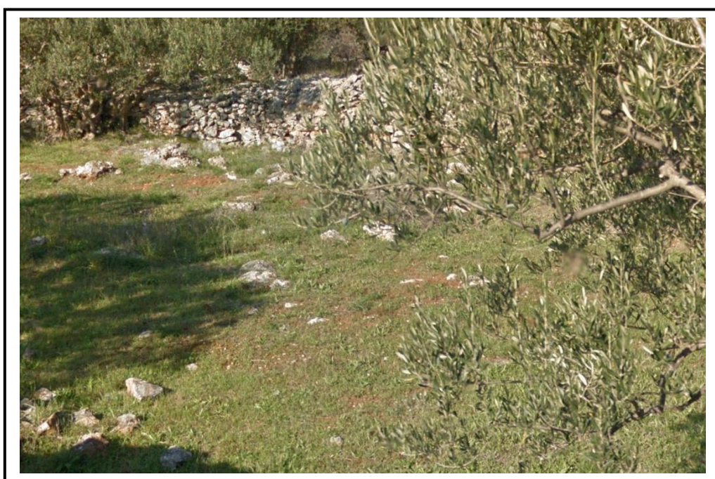
Slike 3 i 4. Matična stijena prekrivena uglavnom tanjim slojem gline uz lokalnu pojavu matične stijene od same površine terena (izdanci stijene)
