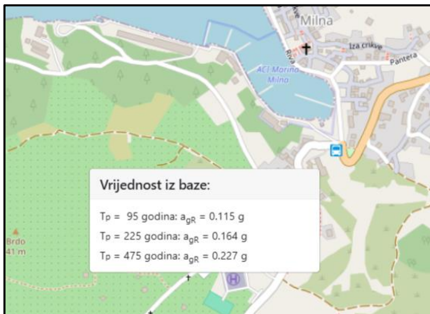
Slika 6. Očitanje iznosa vršnih horizontalnih ubrzanja tla tipa "A" iz karte potresnih područja Republike Hrvatske
