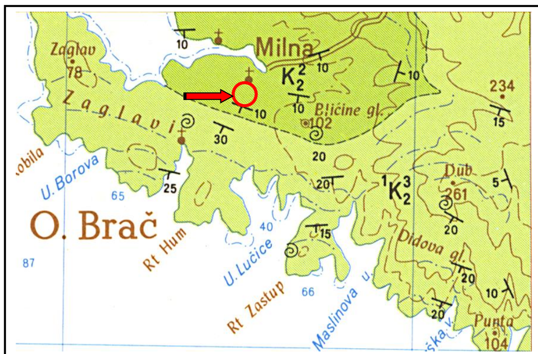
Slika 1. Izvadak iz Osnovne geološke karte Republike Hrvatske - list Vis, M 1:100000 (Autori: I. Borović i dr., IGI - Zagreb, 1967. – 1968.)
