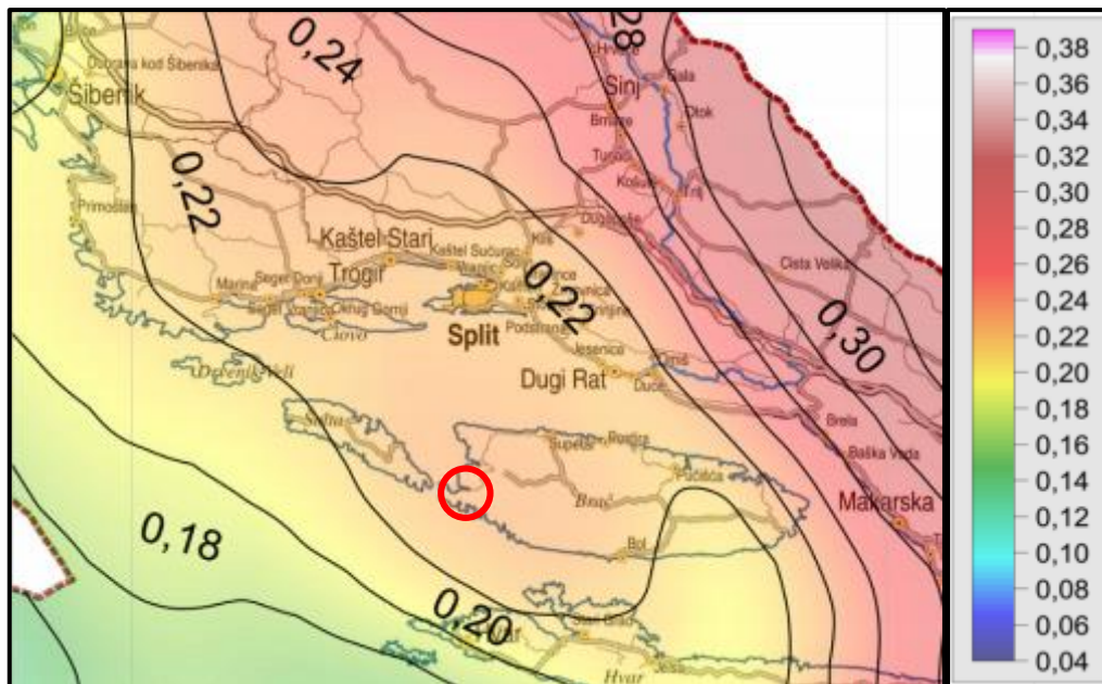
Slika 5. Izvadak iz karte potresnih područja Republike Hrvatske
