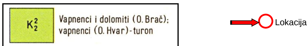
Slika 2. Izvadak iz tumača za Osnovnu Geološku kartu, list Vis
